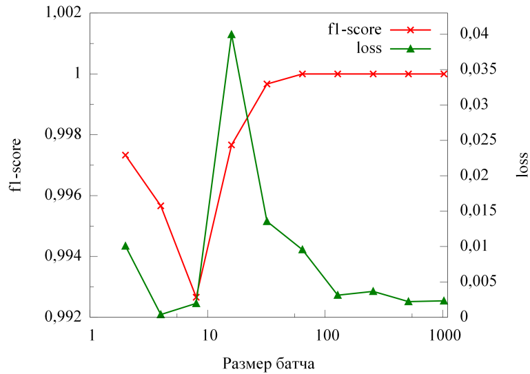
Рис. 1. Зависимость f1-score и loss от размера батча для обучения в течение 1200 итераций
