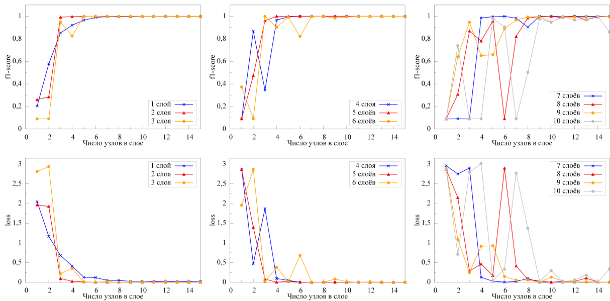
Рис. 3. Зависимость f1-score и loss от количества узлов в сети для тренировочного набора в 10000 элементов
