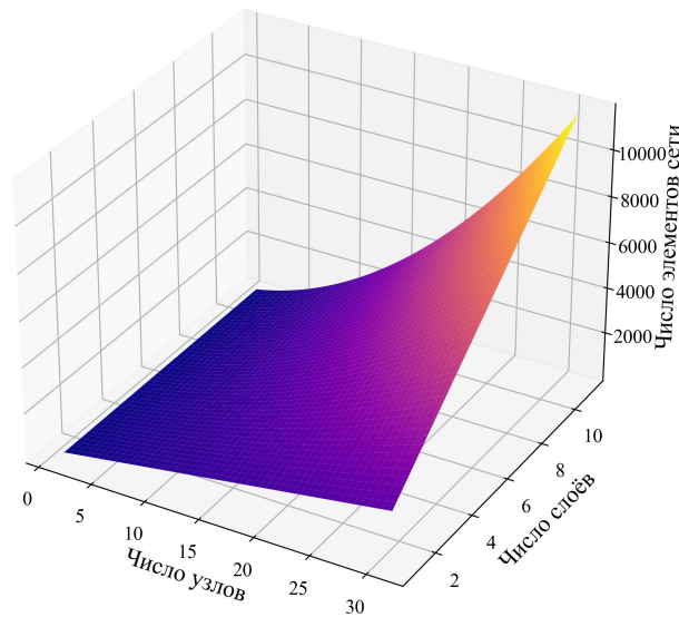
Рис. 2. Зависимость числа оптимизируемых весов от количества узлов и слоёв
