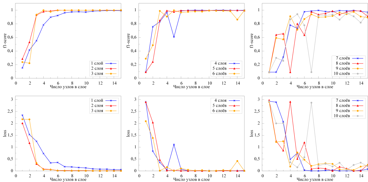
Рис. 4. Зависимость f1-score и loss от количества узлов в сети для тренировочного набора в 1000 элементов
