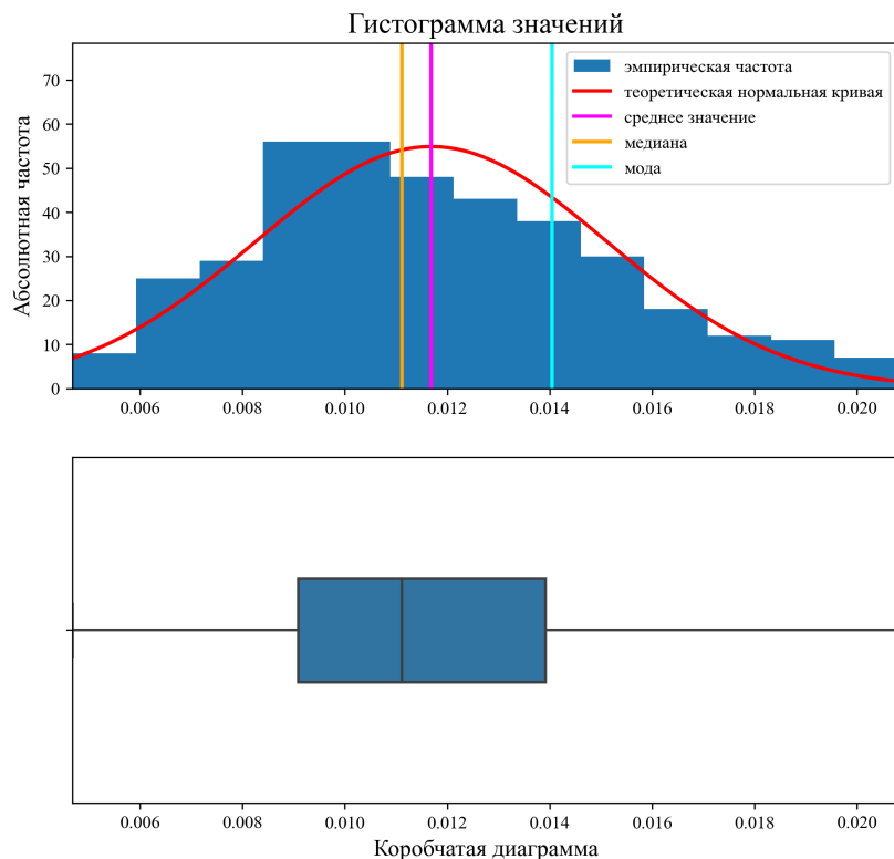
Рис. 5. Гистограмма значений loss и коробчатая диграмма
